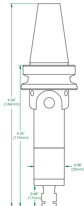
600XBT30 Maße
